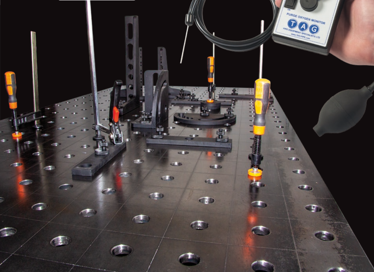
Backinggas- systemen
